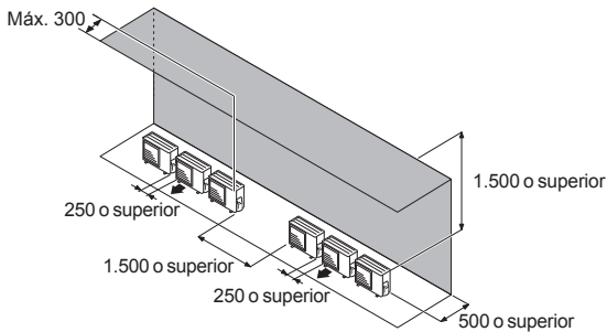
(1) Disposición de la unidad en un paralelo
