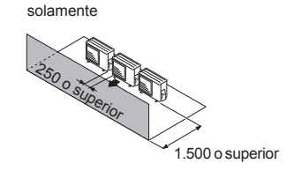
(2) Obstáculos en la parte delantera
