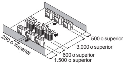
(2) Disposición de la unidad en múltiples paralelos
