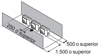
(3) Obstáculos en la parte delantera y posterior
