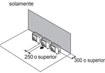
(3) Obstáculos en la parte delantera y posterior
