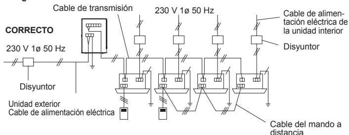
Fig. En caso de unidad exterior conectada
