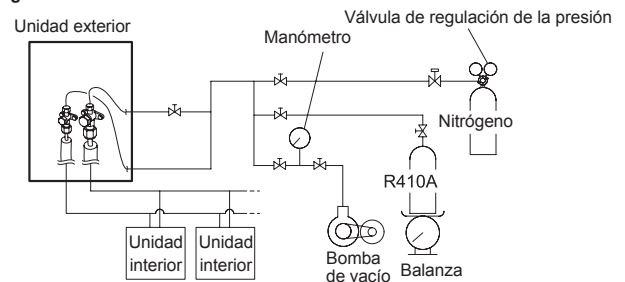
Fig. A Sistema de conexión
