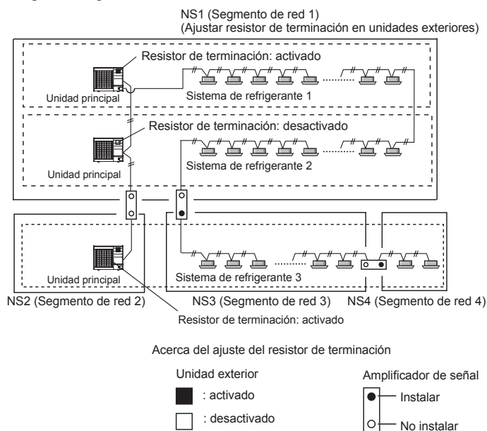
Figura: Configuración del resistor de terminación
